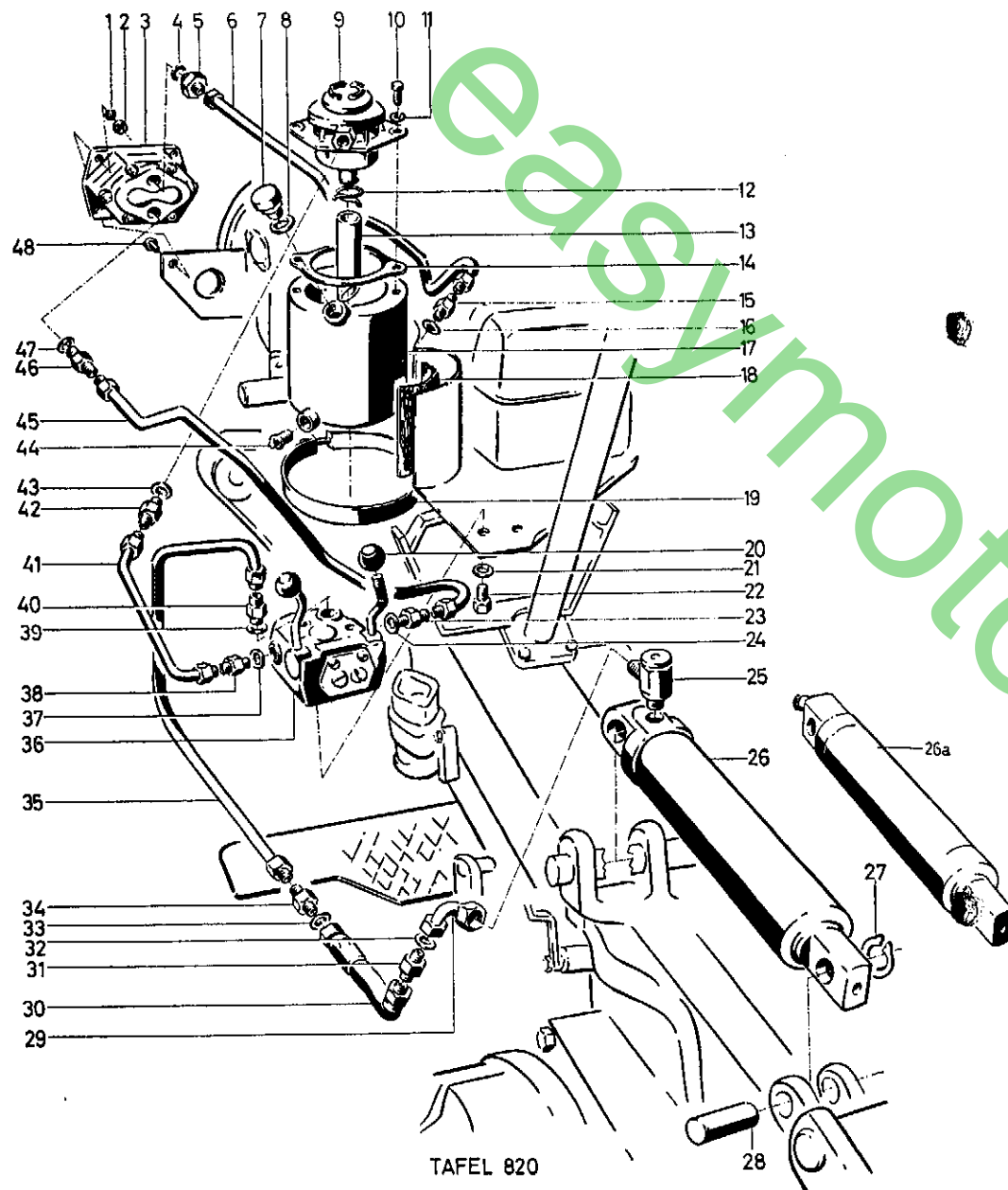
Tafel 820 Hydraulikanlage
