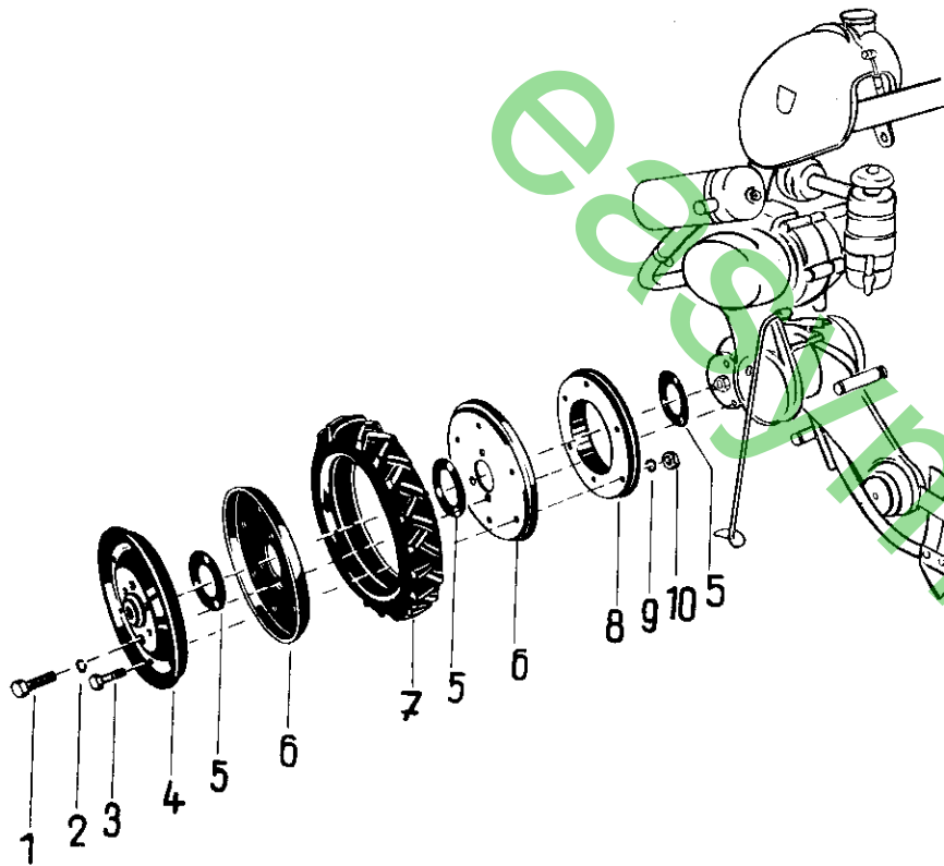
Tafel 372 Laufrad
