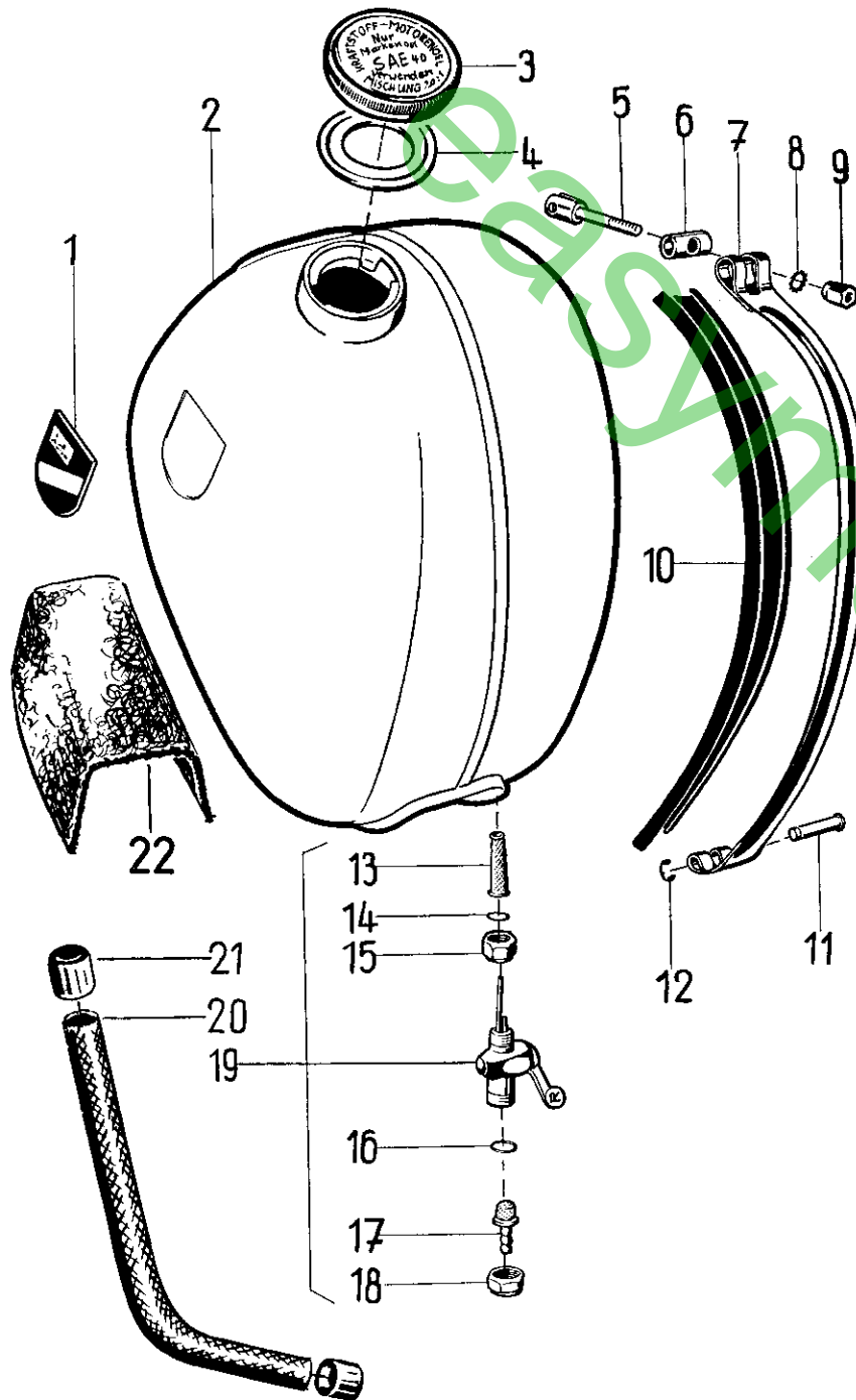
Tafel 349 Kraftstoffbehälter
