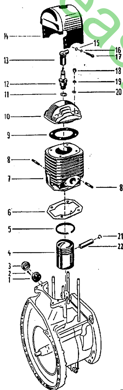
Tafel 281 Zylinder - Kolben (Motor-Typ 34 / 35 M 5 u. 6, 44 / 45 M 5 u. 6)
